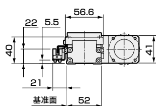
马达相反侧
