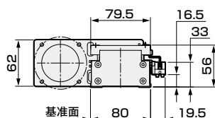
马达相反侧
