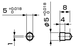
B部详图
