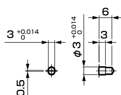
B部详图
