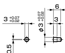
C部详图
