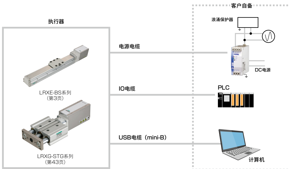
并行I/O (PIO) 连接图
