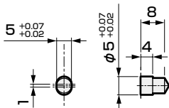
C部详图
